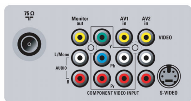
REAR IO
